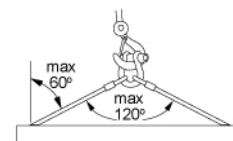
Rys. 3. Maksymalny kąt rozwarcia zawiesi
