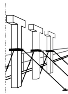
Rys. 4. Stężenia montażowe
